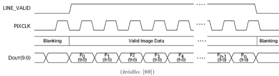
Rysunek 6.2: Transmisja pikseli obrazu.
