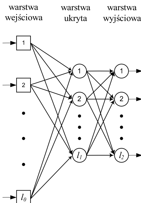
Rysunek 6.14: Struktura sieci neuronowej do rozpoznawania znaków.
