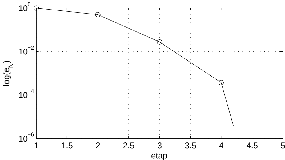
Rysunek 6.24: Wykres metryki Karp-Flatt'a w zrównoleglaniu sieci neuronowej.
